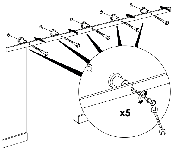
2B Montage op muur van steen/beton - Wand aus Stein/beton Stone/concrete wall - Mur à brique/béton
